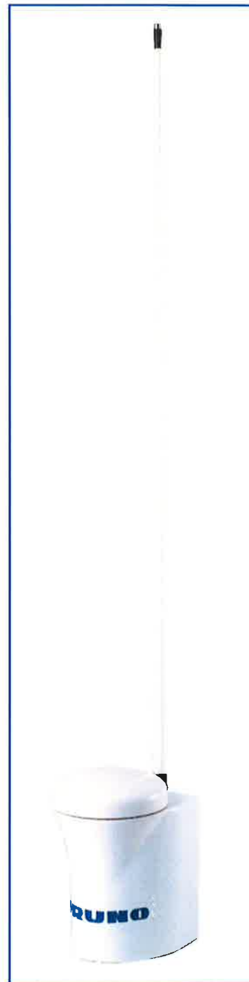
En special GPS/VHF kombinations antenne (GVA-100T) kan købes separat.
